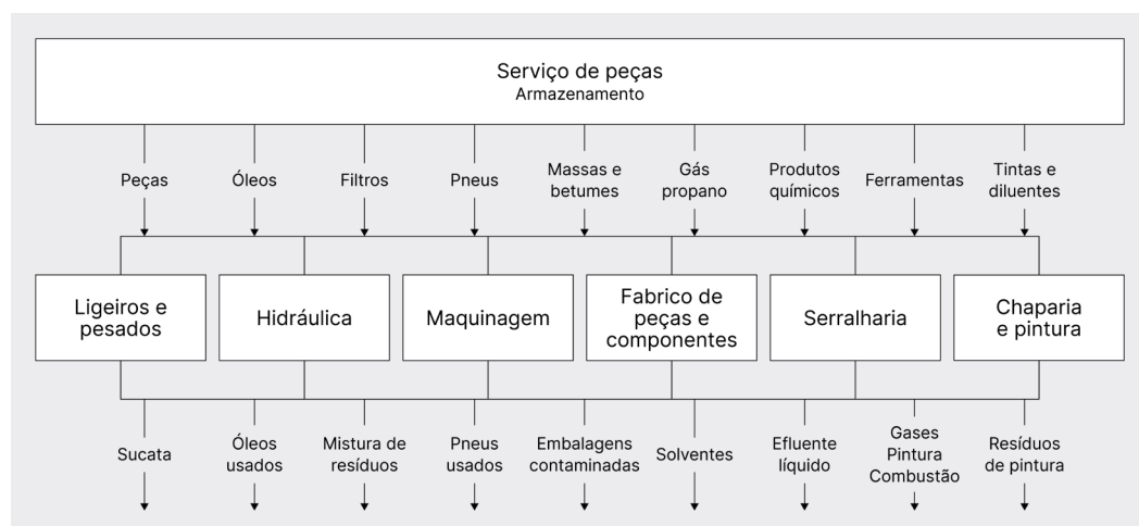
Figura 4. Ciclo produtivo do departamento de manutenção.
